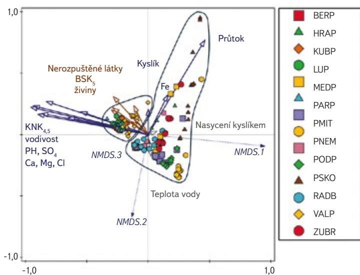
Obr. 3. Analýza NMDS (Canoco 5) pro hodnocené lokality charakterizované měsíčními hodnotami měřených ukazatelů, zobrazena 1. a 2. osa, kumulativní variabilita vysvětlená zobrazenými osami je 94 %
