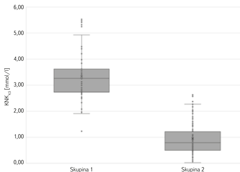
Obr. 4. Krabicový diagram pro ukazatel KNK_{4,5} s rozdělením lokalit do skupin podle analýz PCO a NMDS; skupina 1 = lokality s vyšším obsahem bazických iontů – KNK_{4,5} \geq 2 \text{ mmol/l} , skupina 2 = lokality s nižším obsahem bazických iontů – KNK_{4,5} < 2 \text{ mmol/l}
