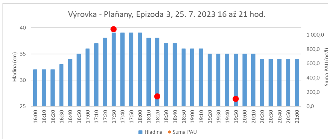
Obr. 6. Koncentrace suma PAU v povrchové vodě během srážkoodtokové epizody č. 3
