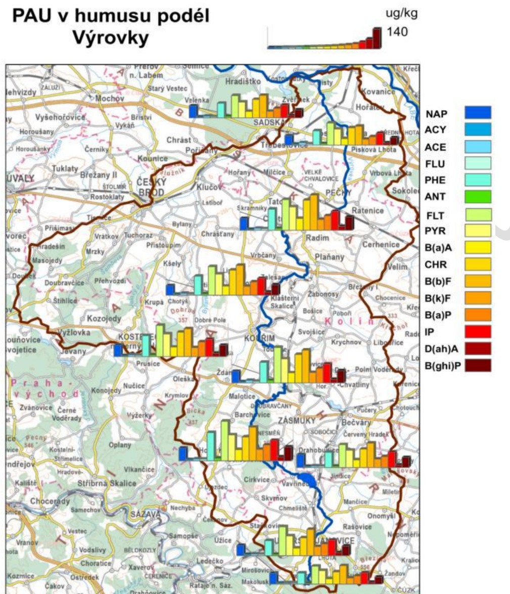
Obr. 11. Rozložení obsahů PAU v lesním humusu v povodí Výrovky v roce 2021
