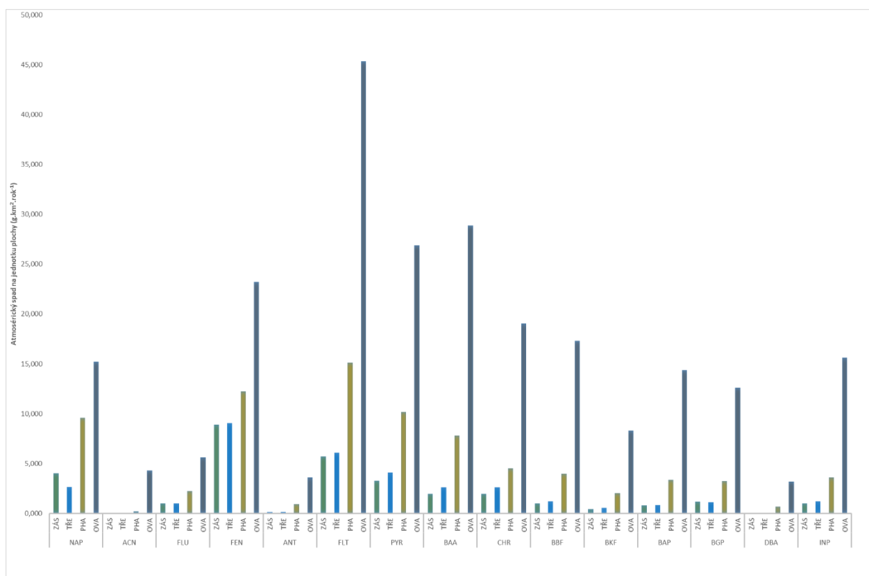
Obr. 8. Porovnání celkového atmosférického spadu PAU na lokalitách Zásmyky, Třebovle, Praha-Podbaba a Ostrava-Přívoz
