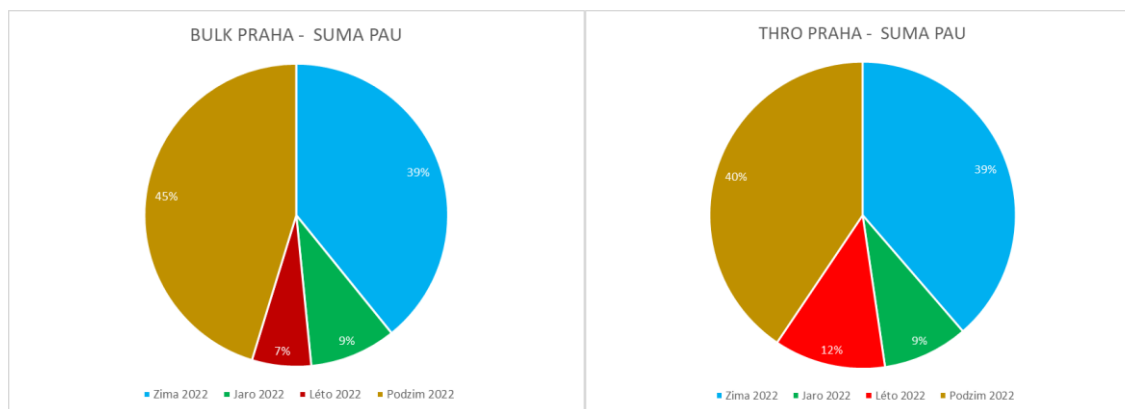
Obr. 9. Poměr sumárních koncentrací PAU ve srážkové vodě podle ročních období v roce 2022, lokalita Praha-VÚV TGM (Podbaba)
