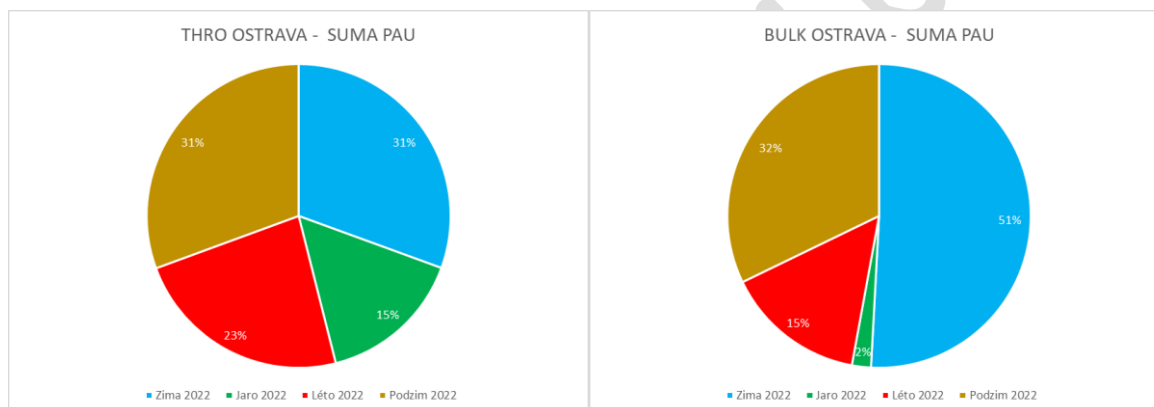
Obr. 10. Poměr sumárních koncentrací PAU ve srážkové vodě podle ročních období v roce 2022, lokalita Ostrava-Privoz
