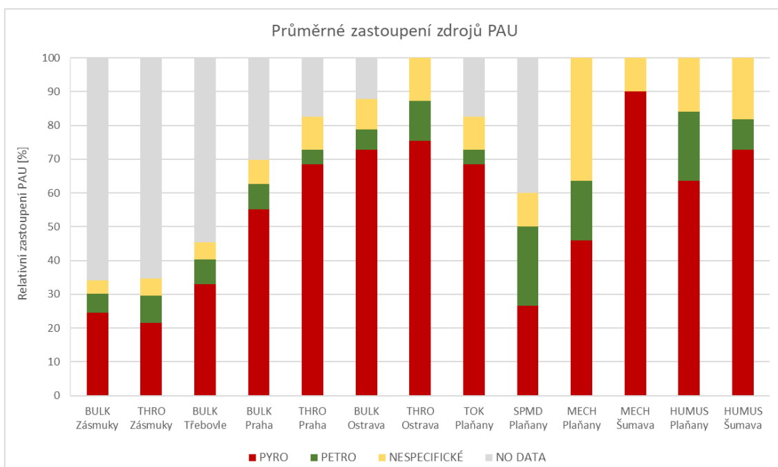
Obr. 13. Průměrné zastoupení zdrojů PAU ve vybraných matricích
