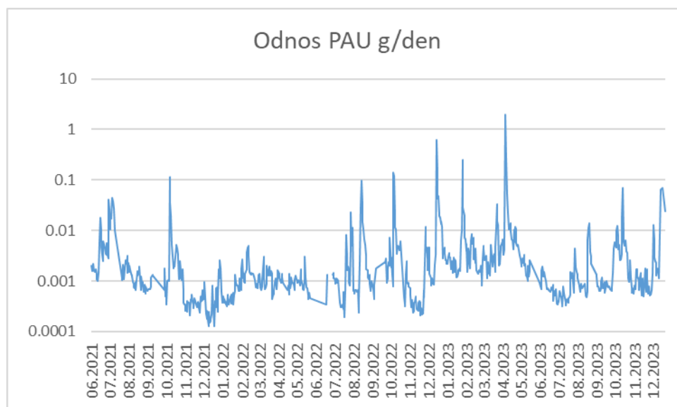
Obr. 5. Režim odnosu PAU v plaveninách v profilu Plaňany v období 2021–2023
