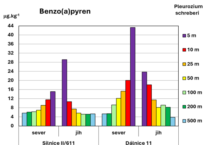
Obr. 12. Pokles obsahu BAP v mechu se vzdáleností od silnice II/611 a dálnice D11 u Sadské v létě roku 2023
