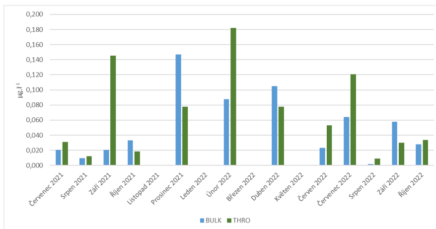
Obr. 2. Suma PAU ve srážkách typu bulk a throughfall na lokalitě Zásmyky
