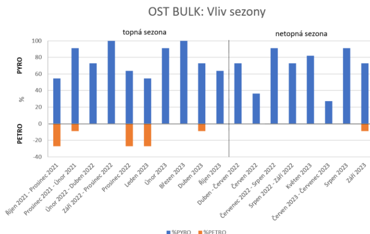
Obr. 15. Původ PAU v mokré atmosférické depozici (bulk) na lokalitě Ostrava
