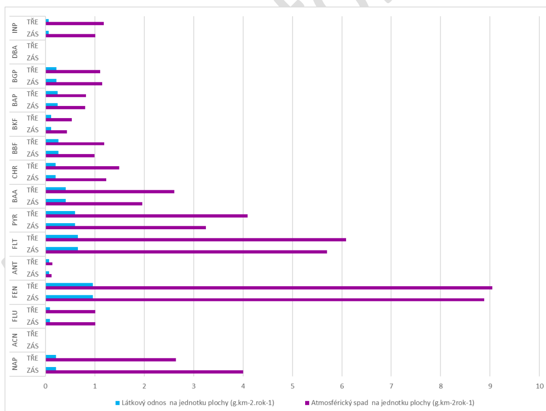
Obr. 4. Celkový atmosférický spad (BULK) PAU na lokalitách Zásmuky a Třebovle a látkový odnos PAU v říčním profilu Výrovka-Plaňany
