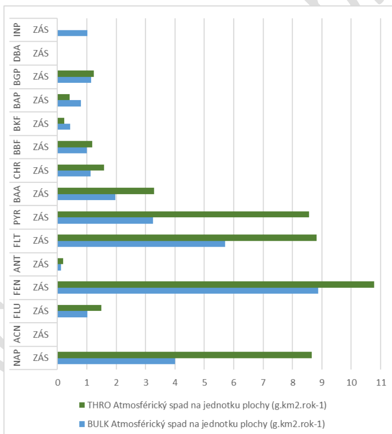
Obr. 3. Atmosférický spad PAU na jednotku plochy depozicí bulk a throughfall na lokalitě Zásmyky
