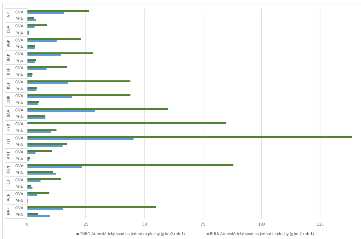
Obr. 7. Srovnání velikosti atmosférického spadu na jednotku plochy ve srážkách typu bulk a throughfall lokalit Ostrava-Přívoz a Praha-Podbaba
