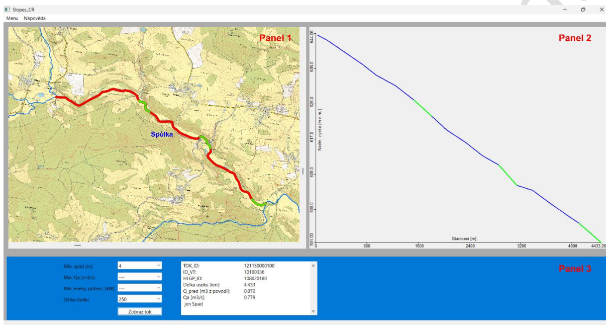
Obr. 4. Identifikace vodních úseků dle nastavených parametrů (panel 1); podélný profil vybraného vodního toku s definovanými úseky (panel 2); a zadané parametry spolu s tabulkovými hodnotami vybraného úseku vodního toku (panel 3)
