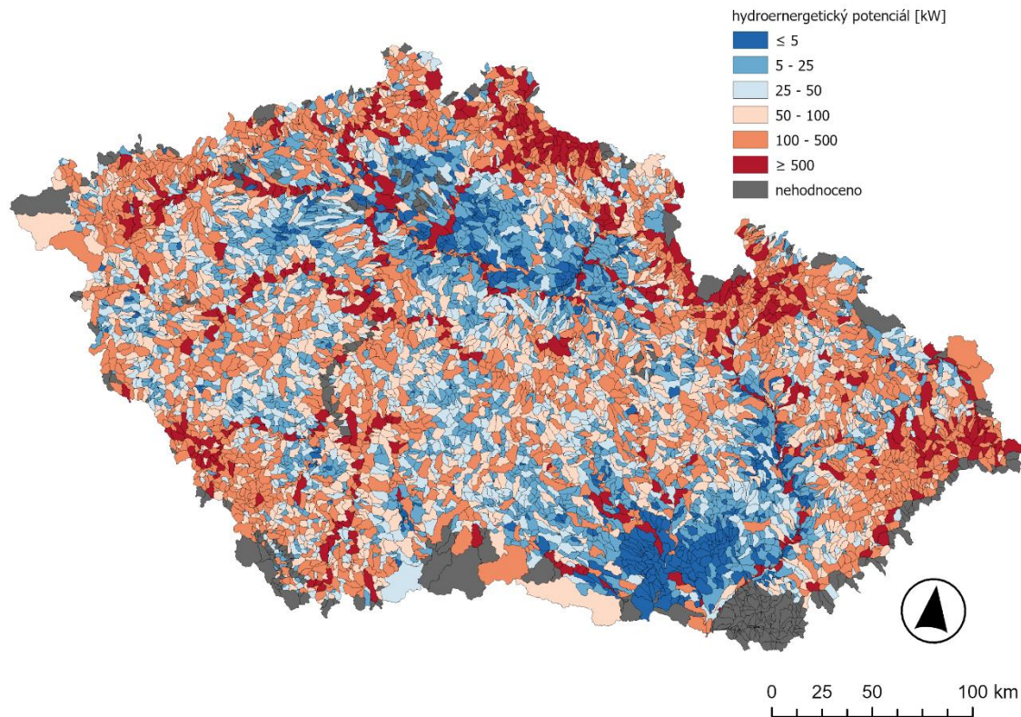
Obr. 3. Odhad teoretického hydroenergetického potenciálu (P) – měřítko povodí IV. řádu
