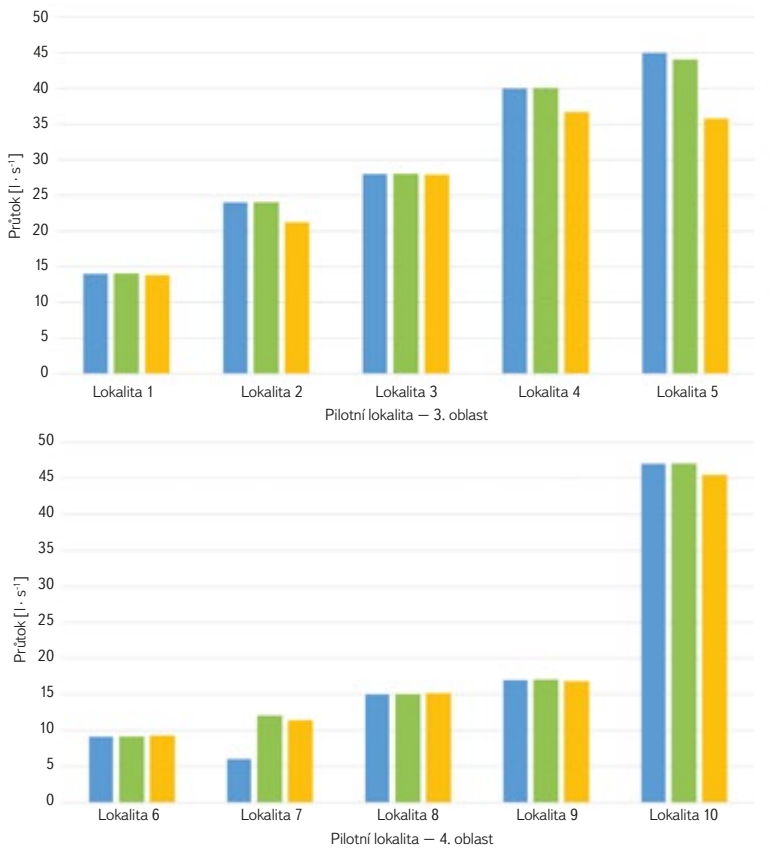
Obr. 2. Porovnání MZP podle návrhu nařízení vlády ve verzi z roku 2019 (žlutý sloupec), dále MZP podle metodického pokynu z roku 1998 (zelený sloupec) a MZP stanoveného v povolení nakládání s vodami (modrý sloupec) pro vybrané lokality ve 3. oblasti a 4. oblasti Fig. 2. Comparison of the MRF according to the draft Regulation of the Government in the 2019 version (yellow column), the MRF according to the Methodical Instruction from 1998 (green column) and the MRF determined in the water management permit (blue column) for selected locations in area 3 and area 4
