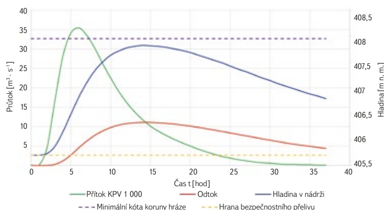
Obr. 7. Průběh transformace povodňové vlny KPV 1 000 ve vodní nádrži
