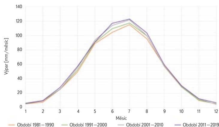
Obr. 5. Ukázka průměrného dekádového měsíčního výparu pro jednu pilotní lokalitu Fig. 5. Example of average decadal monthly evaporation for one pilot site
