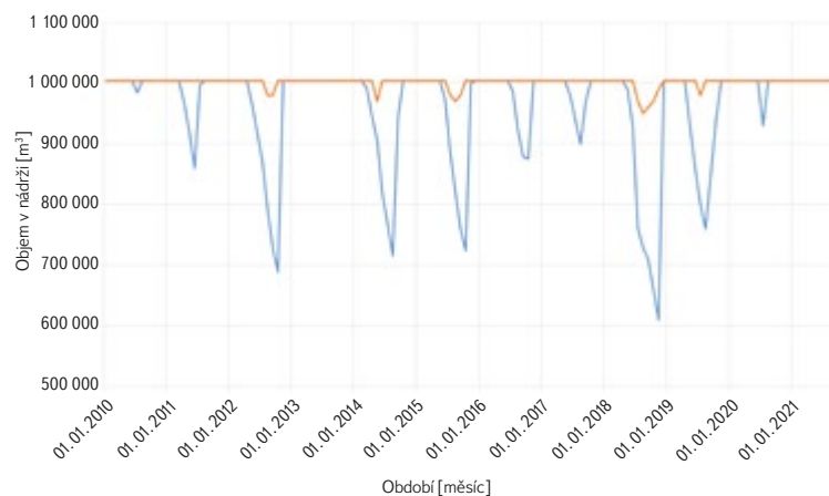
Obr. 6. Ukázka objemu v nádrži při dodržování MZP (modrá křivka) a při nedodržování MZP (oranžová křivka) na odtoku z nádrže za období 2010 až 2021 Fig. 6. Illustration of volume in the reservoir when complying with the MRF (blue curve) and not complying with the MRF (orange curve) at the reservoir outlet for the period from 2010 to 2021
