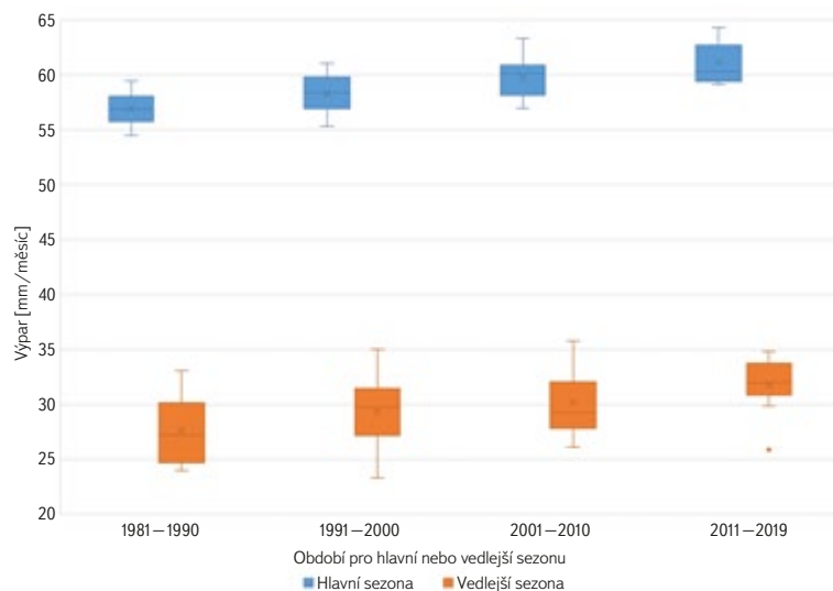
Obr. 4. Ukázka průměrného dekádového výparu pro hlavní sezona a vedlejší jarní sezona pro jednu pilotní lokalitu Fig. 4. Example of average decadal evaporation for the main season and for the secondary spring season for one pilot site
