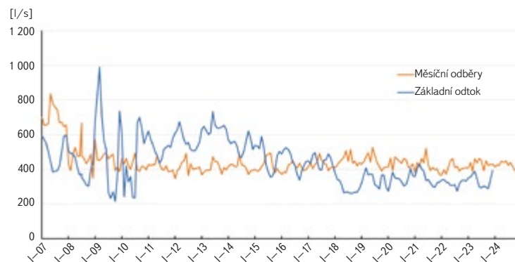
Obr. 9. Zpracování vodohospodářské bilance v měsíčním kroku – období 2007–2024 [17, 18] Fig. 9. Water management balance in a monthly step, 2007–2024 [17, 18]
