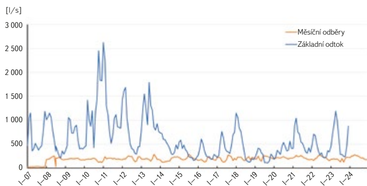
Obr. 7. Zpracování vodohospodářské bilance v měsíčním kroku – období 2007–2024 [17, 18] Fig. 7. Water management balance in a monthly step, 2007–2024 [17, 18]
