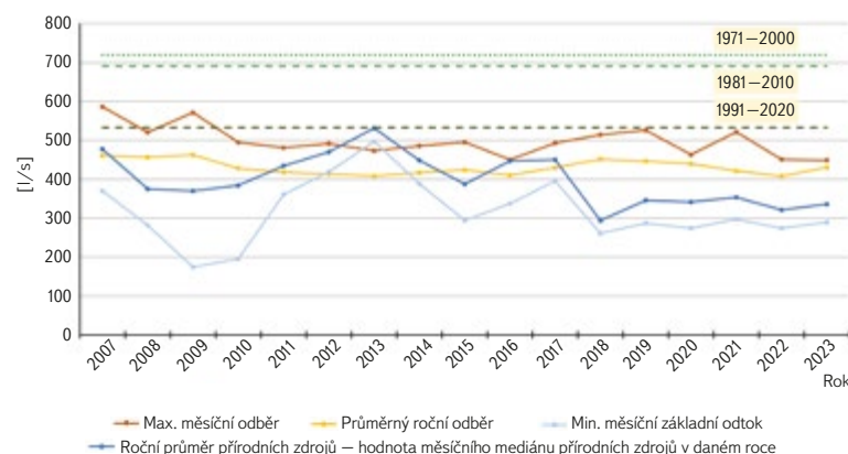
Obr. 8. Roční charakteristiky pro základní bilanční hodnocení HGR 4522 včetně dlouhodobého charakteristického období 1971–2000, 1981–2010 a 1991–2020 Fig. 8. Annual characteristics for basic balance assessment of HGR 4522, including long-term reference periods 1971–2000, 1981–2010, and 1991–2020
