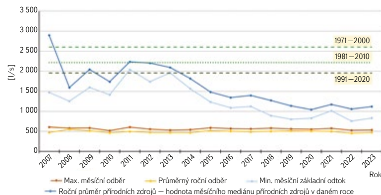
Obr. 4. Roční charakteristiky pro základní bilanční hodnocení HGR 4410 včetně dlouhodobého charakteristického období 1971–2000, 1981–2010 a 1991–2020
