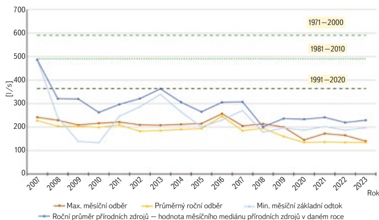
Obr. 10. Roční charakteristiky pro základní bilanční hodnocení HGR 4523 včetně dlouhodobého charakteristického období 1971–2000, 1981–2010 a 1991–2020
