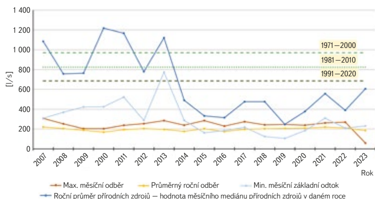
Obr. 6. Roční charakteristiky pro základní bilanční hodnocení HGR 4430 včetně dlouhodobého charakteristického období 1971–2000, 1981–2010 a 1991–2020 Fig. 6. Annual characteristics for basic balance assessment of HGR 4430, including long-term reference periods 1971–2000, 1981–2010, and 1991–2020
