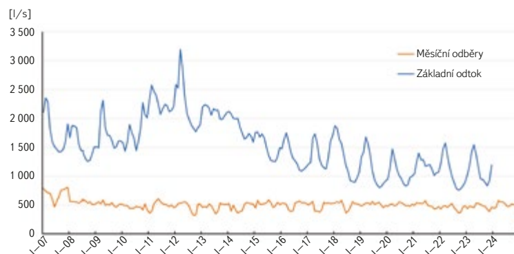
Obr. 5. Zpracování vodohospodářské bilance v měsíčním kroku – období 2007–2023 [17, 18] Fig. 5. Water management balance in a monthly step, 2007–2023 [17, 18]
