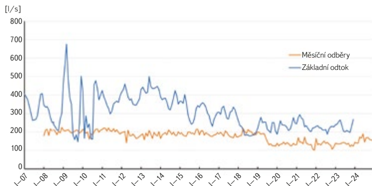
Obr. 11. Zpracování vodohospodářské bilance v měsíčním kroku – období 2007–2024 [17, 18]
