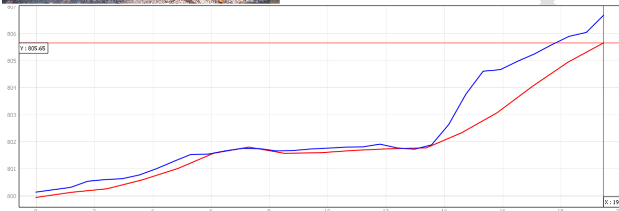
Obr. 2a, b. Příčný profil cesty odvozený z DMR z leteckého laserového skenování s rozlišením 1 m (červeně, Správa KRNAP) a 50 cm (modře, ČVUT) pro testování identifikace terénní konfigurace cesty a výskytu prvků podélného odvodnění; nahore fotografie skutečného stavu z terénního průzkumu
