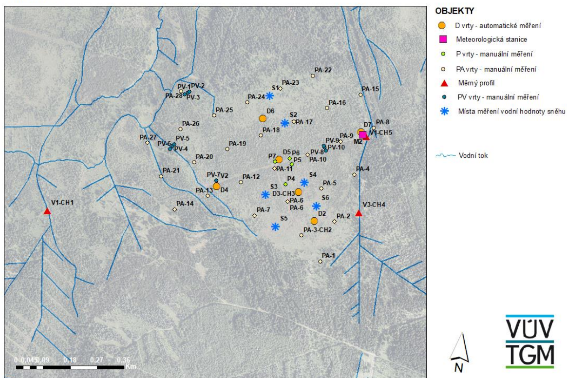
Obr. 2 [ZŘ2]. [ZŘ3] Objekty monitoringu v ploše A
