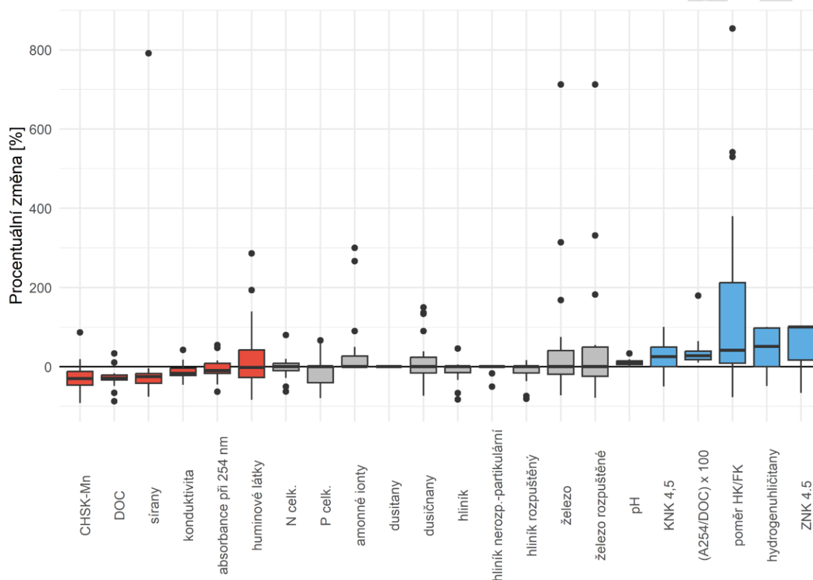
Obr. 7. Krabicové grafy procentuálních změn obsahu látek mezi profily CH9 nad nádrží a CH10 pod nádrží; hlavní částí je „krabice“ mezi prvním a třetím kvantilem, uvnitř níž je čára označující median; z krabice vycházejí „vousy“, jež zobrazují rozsah dat mimo kvantily (typicky až 1,5násobek interkvartilního rozpětí); odlehlé hodnoty jsou zobrazovány jako samostatné body mimo vousy
