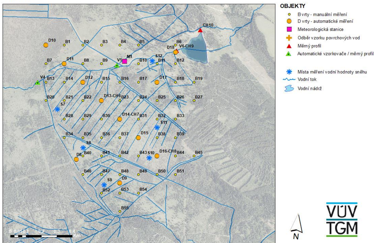
Obr. 3. Objekty monitoringu v ploše B
