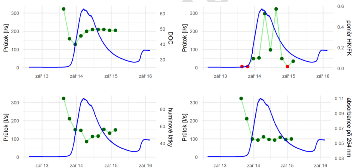
Obr. 6. [ZŘ5] Výsledky automatického vzorkování významné srážkoodtokové události 13. až 15. září 2025 na profilu V5
