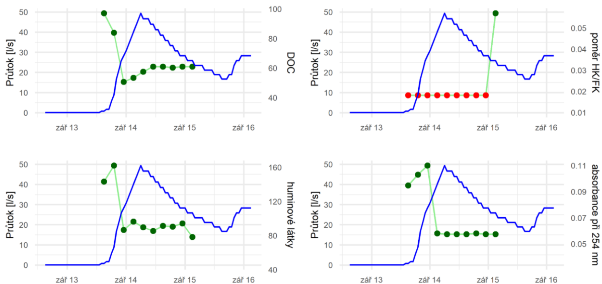
Obr. 5. [ŘZ4] Výsledky automatického vzorkování významné srážkoodtokové události 13. až 15. září 2024 na profilu V4
