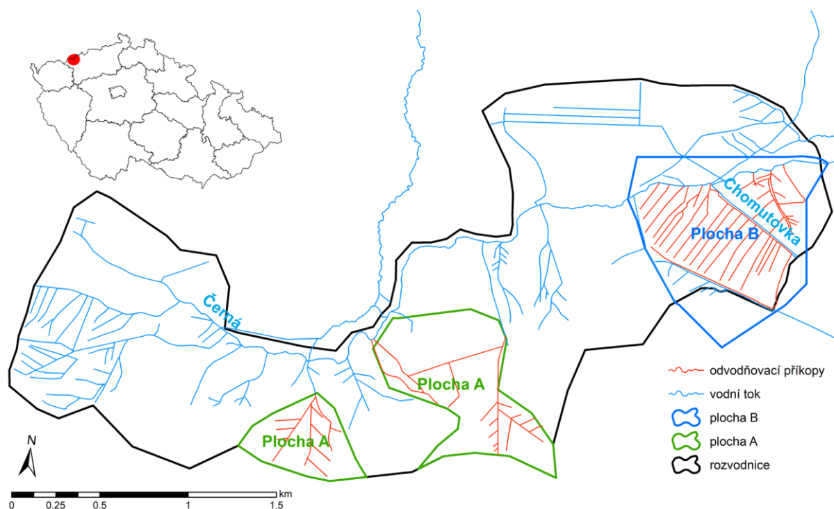
Obr. 1. [ŘZ1]Schéma monitorovacích ploch A a B (plocha A vlevo odpovídá rozvodnici pro profil V1-CH1, viz obr. 2); rozvodnice vodního toku Chomutovka v řadě případů nerespektuje sklonové poměry povodí díky odvodňovacím kanálům, proto je rozvodnice do jisté míry založena na terénním průzkumu a následném expertním odhadu
