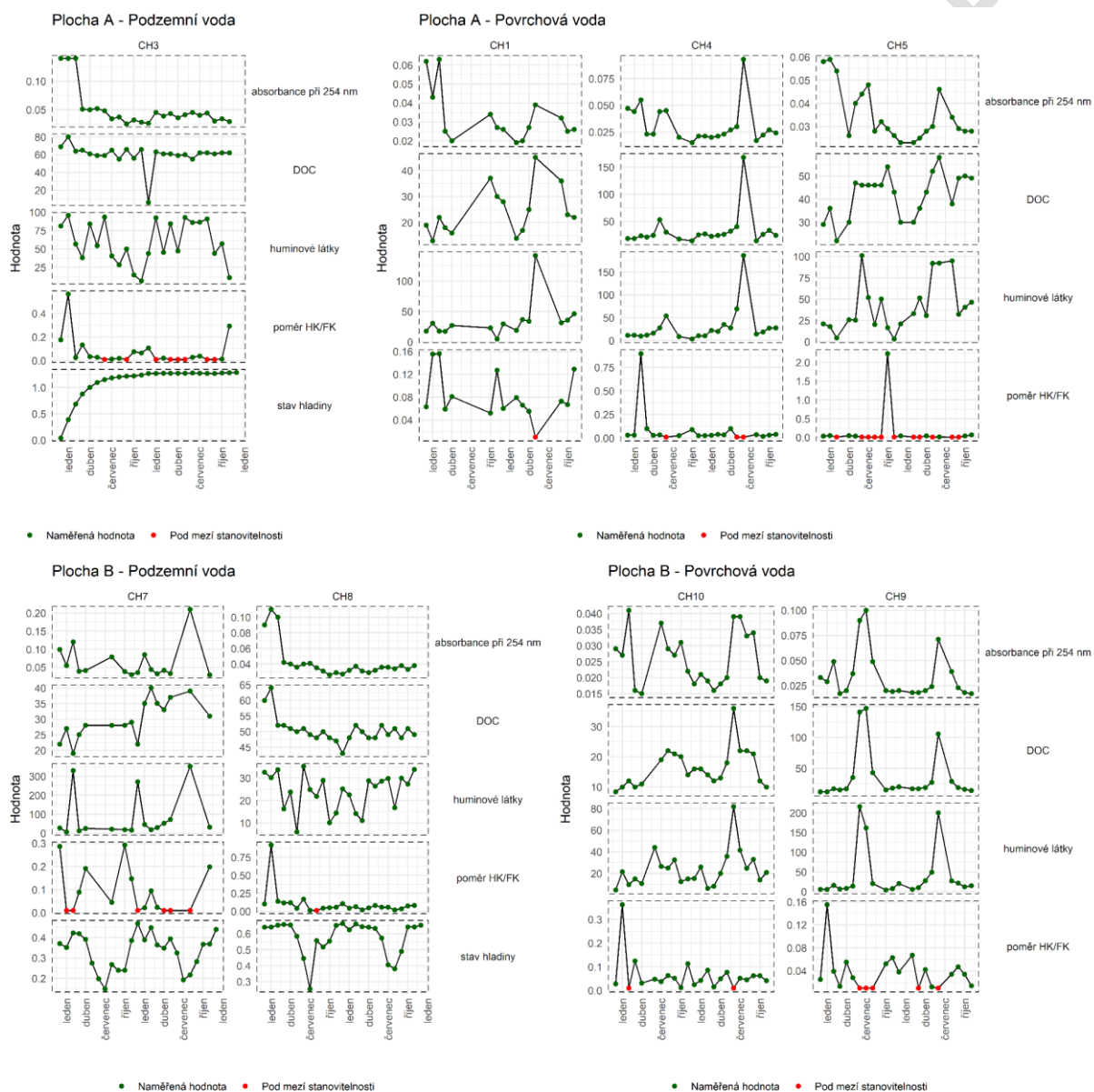
Obr. 4. Výsledky chemických rozborů vybraných ukazatelů
