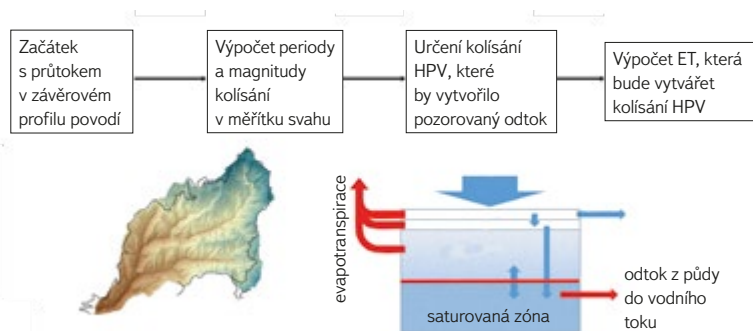
Obr. 4. Schematický přehled Fonleyova postupu zpětného výpočtu ET ze záznamu diurnálního kolísání průtoku ve vodním toku (upraveno podle [13])
