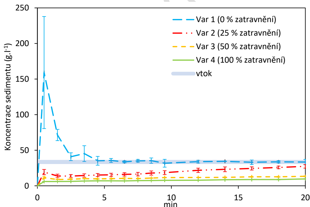
Obr. 4. Průběh koncentrace povrchového odtoku testovaných variant 1–4. Jde o průměrné hodnoty ze tří replikací pro každou variantu; chybové úsečky reprezentují směrodatnou odchylku jednotlivých replikací
