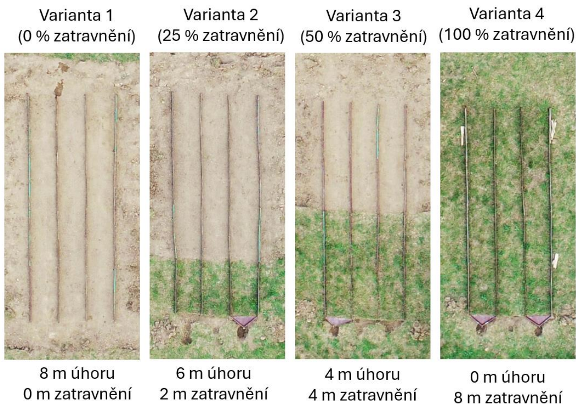
Obr. 2. Ortofoto snímky experimentálních ploch testovaných variant 1–4
