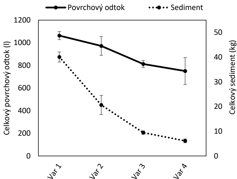
Obr. 5. Celkové množství povrchového odtoku a sedimentu variant 1–4. Jde o průměrné hodnoty ze tří replikací pro každou variantu; chybové úsečky reprezentují směrodatnou odchylku jednotlivých replikací
