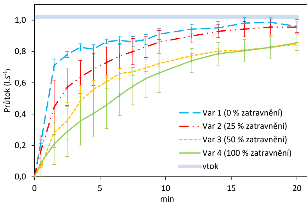
Obr. 3. Průběh povrchového odtoku testovaných variant 1–4. Jde o průměrné hodnoty ze tří replikací pro každou variantu; chybové úsečky reprezentují směrodatnou odchylku jednotlivých replikací
