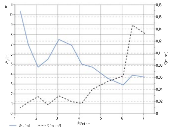
Obr. 3. a) Poproudový vývoj zrnitosti sedimentů D_{25} , D_{50} , D_{95} a SPI; b) poproudový vývoj šířek ( W_{cr} ) a sklonů ( S ) hlavního koryta Slavíče Fig. 3. a) Downstream grain size trends of sediments D_{25} , D_{50} , D_{95} and SPI; b) downstream trends of width ( W_{cr} ) and slope ( S ) of the Slavice channel
