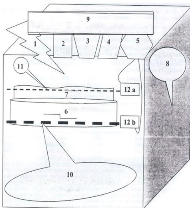
Obr. 1. Schéma zařízení pro fyzikální předúpravu odpadu
