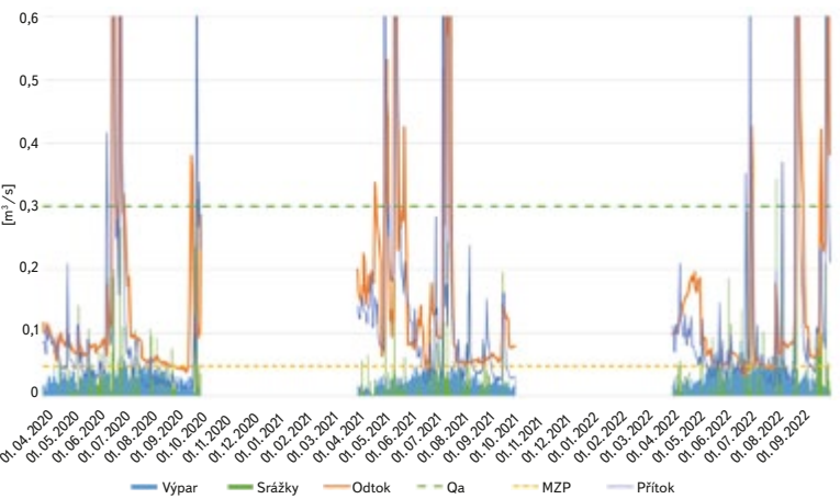
Obr. 6. Výpar z vodní plochy ve srovnání se srážkami, přítokem a odtokovými charakteristikami Vavříneckého rybníka 1. duben 2020 – 30. září 2022 Fig. 6. Volume of water level evaporation compared to the precipitation, inflow and water outflow characteristics at Vavřínek pond 1st April 2020 – 30th September 2022
