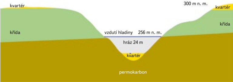
Obr. 6. Schematizovaný převýšený geologický řez lokalitou LAPV Tucharaz na Šemberě Fig. 6. Schematic geological exaggerated section of locality LAPV Tucharaz, Šembera stream
