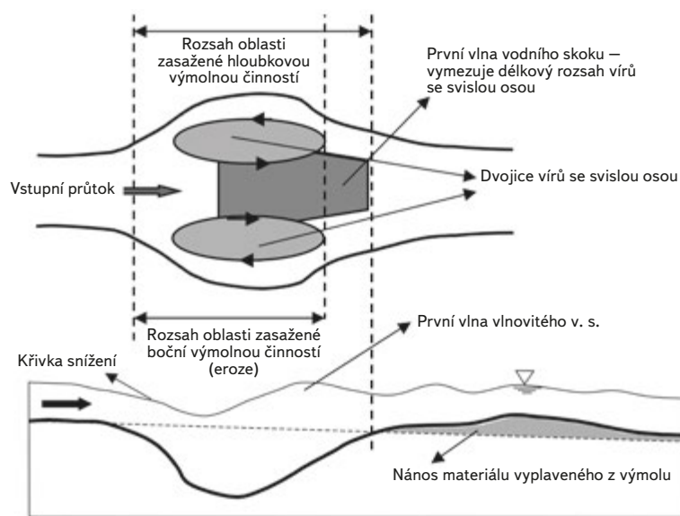
Obr. 1. Vývoj „výmolu – hrušky“ iniciovaného porušením spádového stupně při povodni (vlevo); schematické naznačení charakteru proudění v přechodové oblasti prostorového výmolu (vpravo) Fig. 1. Development of the “pear shaped” scour resulting from degradation of a drop structure on flash flood occurrence (left); feature of flow in transitional zone of the spatial 3D scour (right)
