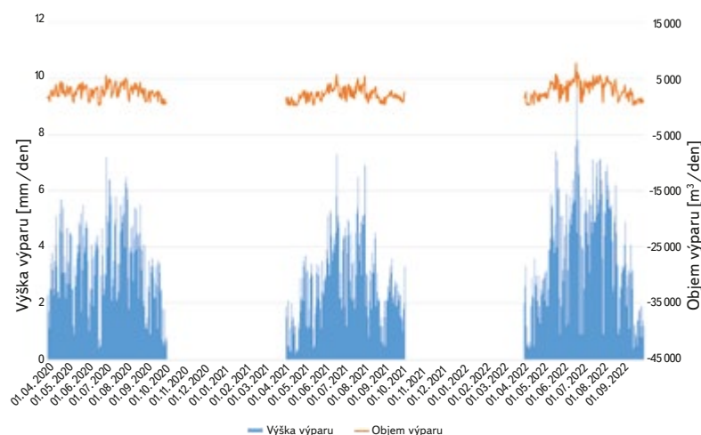
Obr. 5. Výpar z vodní plochy Vavříneckého rybníka v období 1. duben 2020 – 30. září 2022
