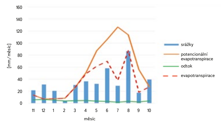
Obr. 7. Průběh bilančních hydrologických veličin v roce 2015 – povodí Rakovnického potoka
