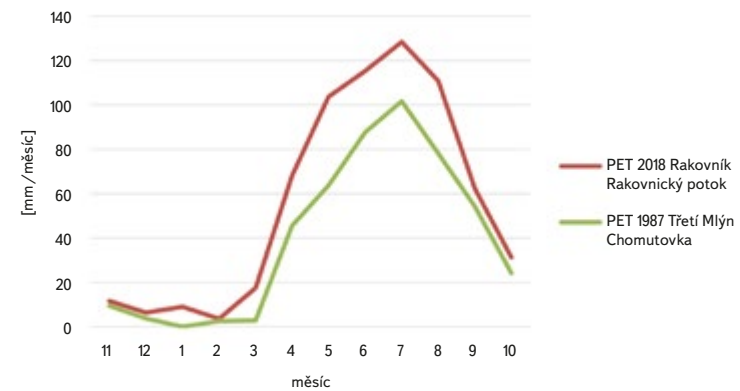
Obr. 3. Průběh potenciální evapotranspirace (PET) v teplém roce 2018 na povodí Rakovnického potoka a chladném roce 1987 na povodí Chomutovky
