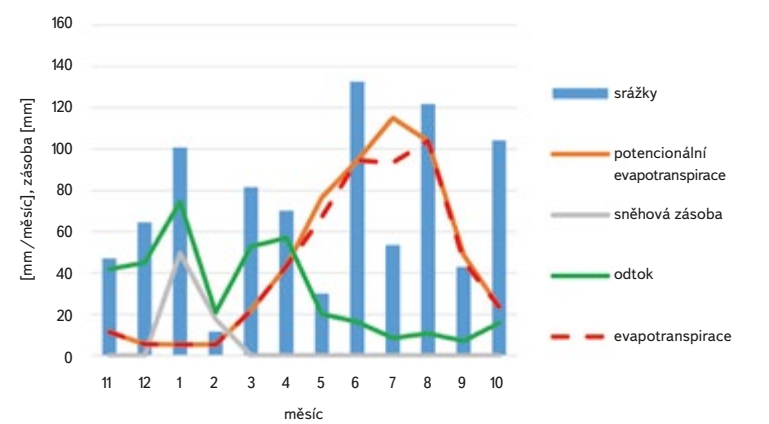
Obr. 5. Průběh bilančních hydrologických veličin v roce 2015 – povodí Chomutovky
