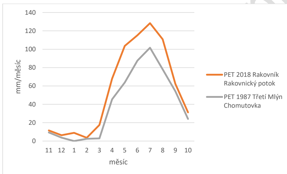
Obr. 3. Průběh potenciální evapotranspirace (PET) v teplém roce 2018 na povodí Rakovnického potoka a chladném roce 1987 na povodí Chomutovky
