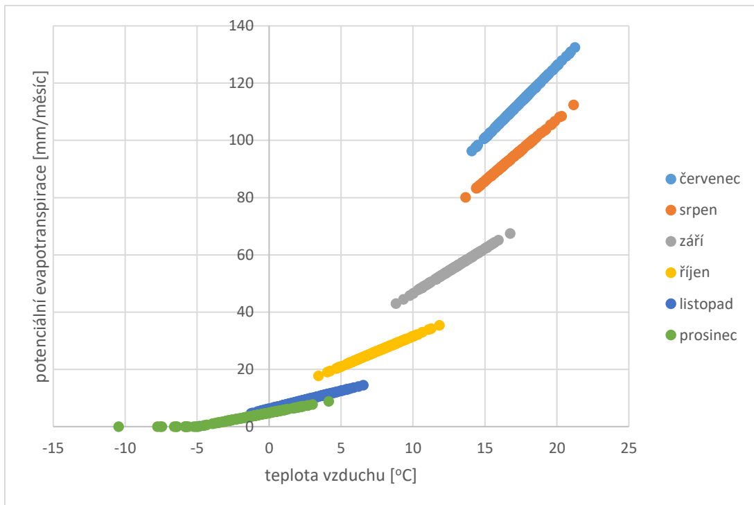
Obr. 10 [BH3]. Vztah mezi teplotou a potenciální evapotranspirací v jednotlivých měsících 2. pololetí
