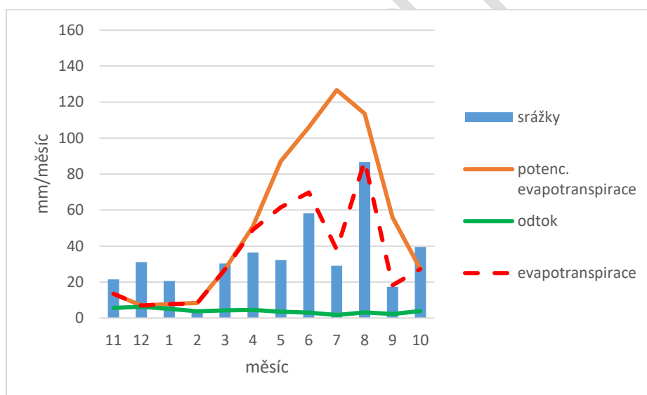
Obr. 7. Průběh bilančních hydrologických veličin v roce 2015 – povodí Rakovnického potoka
