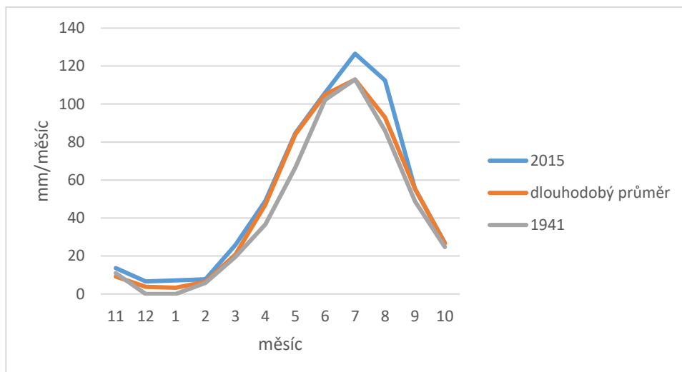
Obr. 2. [ŘZ1] Průběh potenciální evapotranspirace na povodí Labe po Děčín v teplém roce 2015, v extrémně chladném roce 1941 a v dlouhodobém průměru
