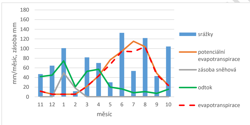
Obr. 5. Průběh bilančních hydrologických veličin v roce 2015 – povodí Chomutovky
