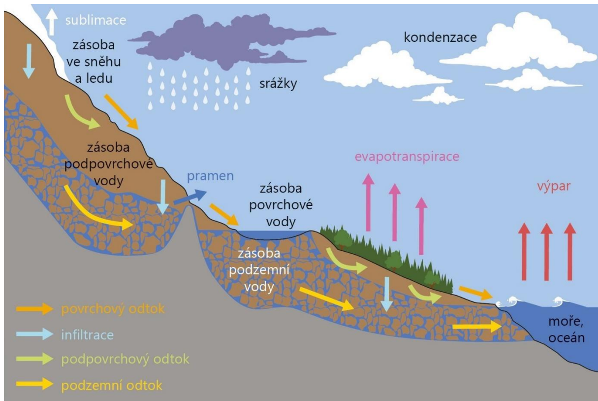
Obr. 1. Schéma hydrologického cyklu [2]
