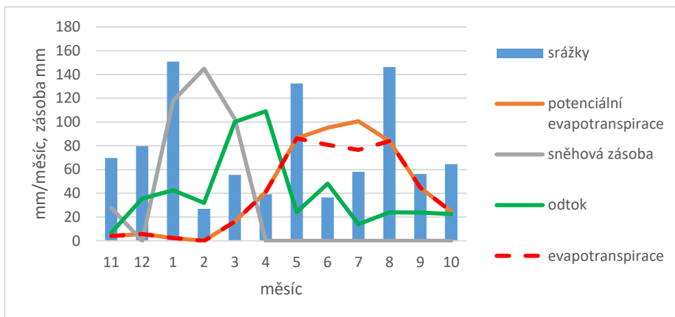
Obr. 4. Průběh bilančních hydrologických veličin v roce 1986 – povodí Chomutovky
