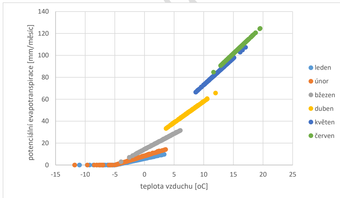
Obr. 9. [Ř22] Vztah mezi teplotou a potenciální evapotranspirací v jednotlivých měsících 1. pololetí
