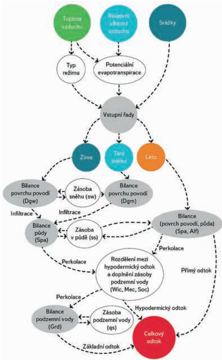
Obr. 1. Schéma popisující strukturu modelu BILAN v měsíčním výpočetním kroku
