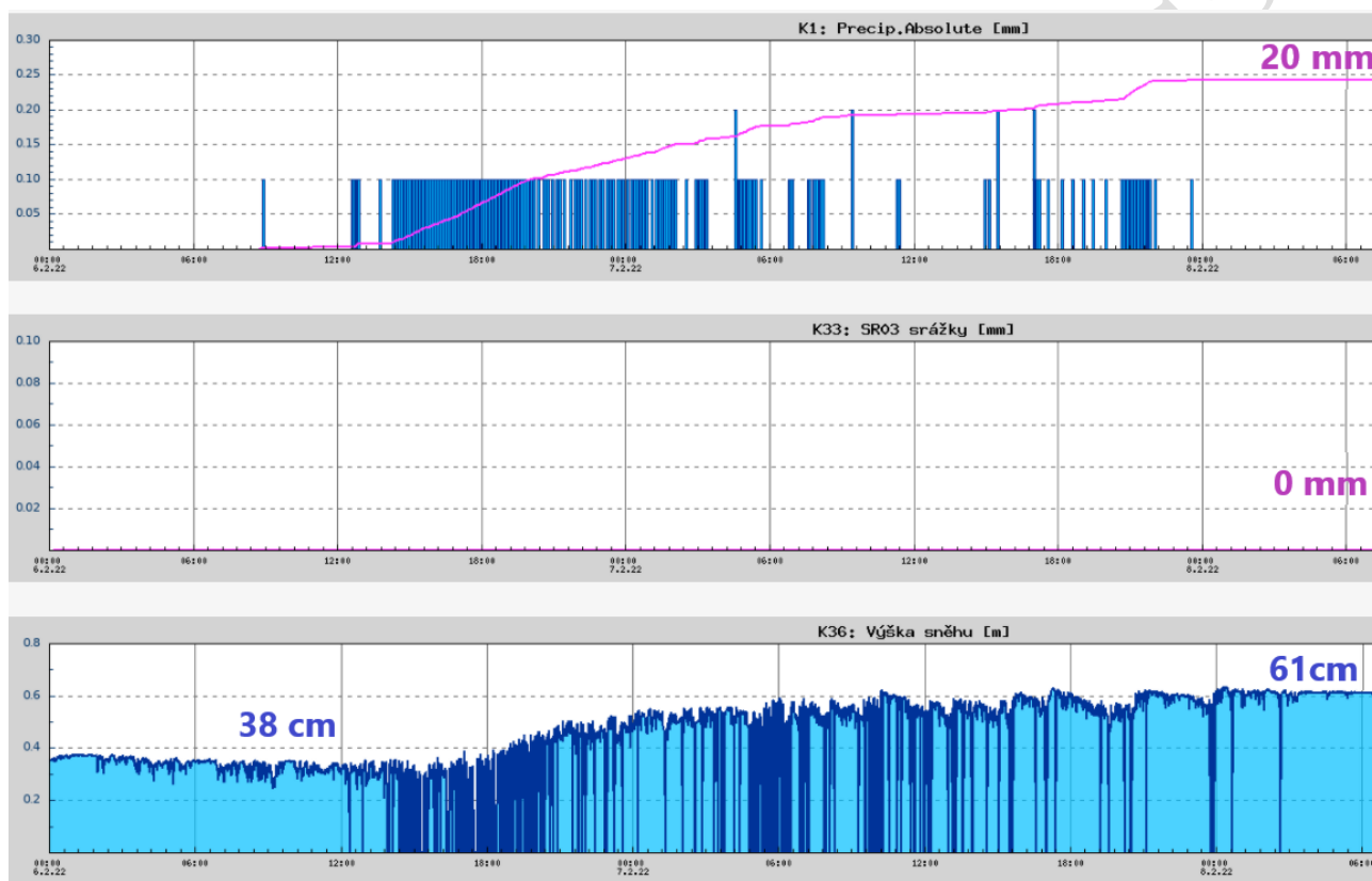
Obr. 4. Výstupy radarového srážkoměru WS100 (první graf), nevyhřívávaného člunkového srážkoměru SR03 (druhý graf) a ultrazvukového měření výšky sněhu (třetí graf) během vydatného sněžení 6.–7. února 2022
