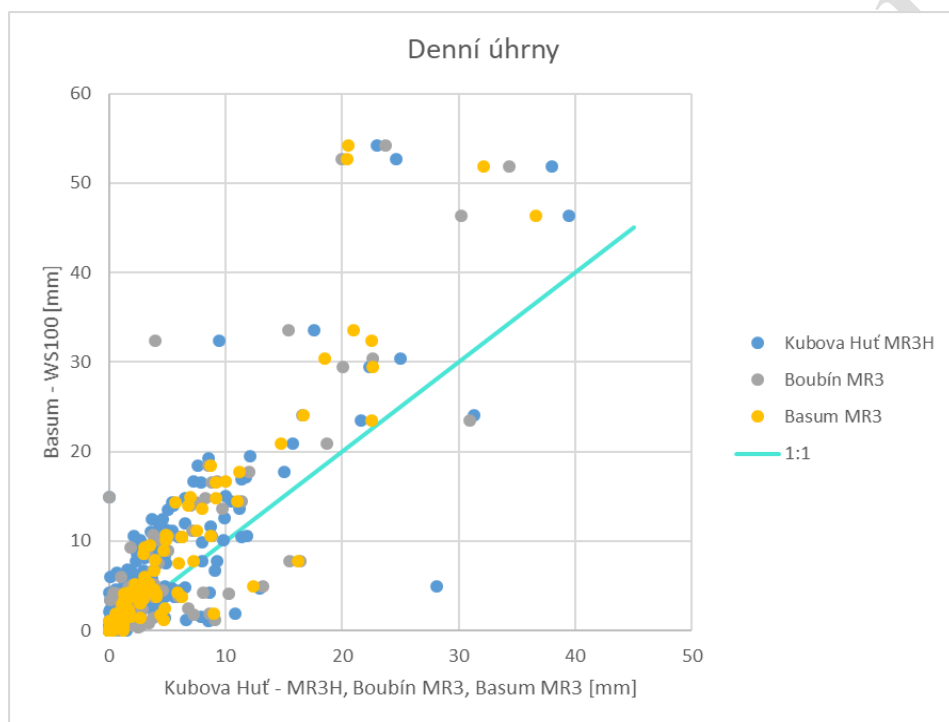
Obr. 8. Srovnání denních úhrnů v hydrologickém roce 2021 měřených radarovým srážkoměrem WS100, nejbližšími meteorologickými stanicemi Kubova Huť, Boubín a člunkovým srážkoměrem na stanici Basum
