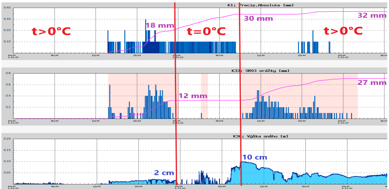
Obr. 6. Výstupy radarového srážkoměru WS100 (první graf), nevyhříváného člunkového srážkoměru SR03 (druhý graf) a ultrazvukového měření výšky sněhu (třetí graf). Červené svislice oddělují časový úsek, kdy teplota klesla na bod mrazu. Číselně jsou uvedeny dílčí sumy srážek a výšky sněhu
