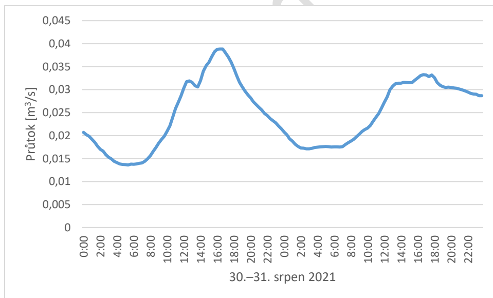
Obr. 7. Denní chod odtoku z povodí (ukázka dat pro 30. a 31. srpen 2021)
