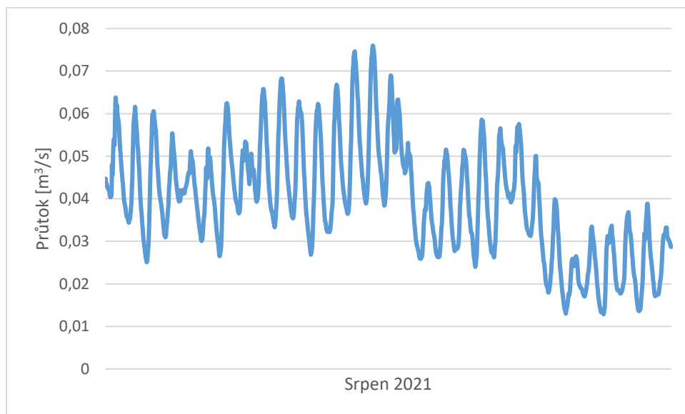
Obr. 6. Rozkolísanost průtoků po realizaci revitalizace (ukázka dat ze srpna 2021)
