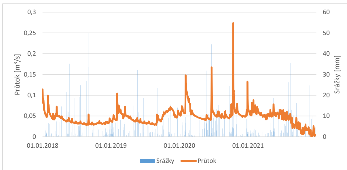
Obr. 5. Průtok a srážky v období od 1. ledna 2018 do 31. prosince 2021
