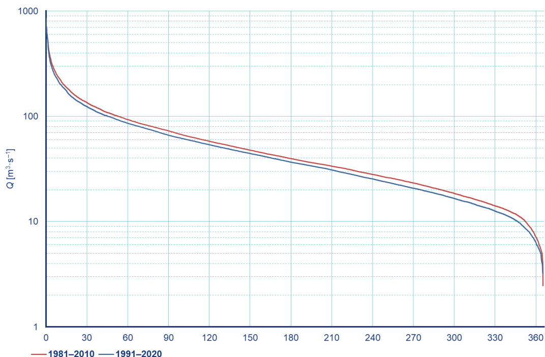
Obr. 7. Čáry překročení M -denních průtoků v období 1981–2010 a v období 1991–2020 v profilu vodoměrné stanice Strážnice na Moravě
