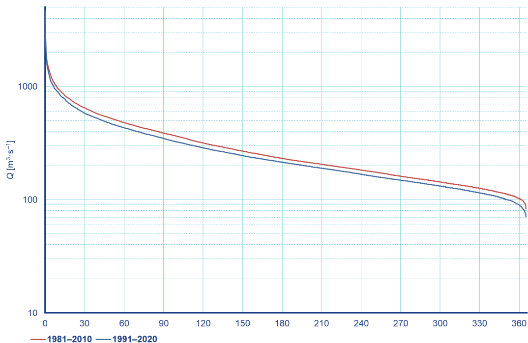
Obr. 5. Čáry překročení M -denních průtoků v období 1981–2010 a v období 1991–2020 v profilu vodoměrné stanice Děčín na Labi
