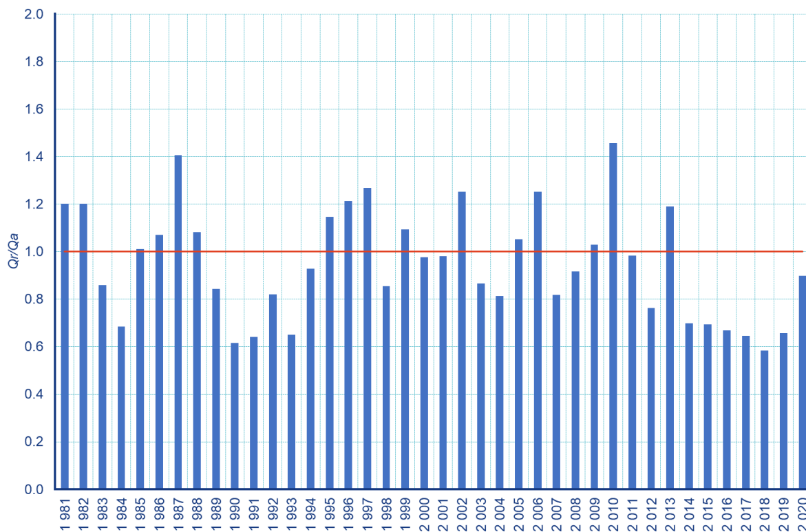
Obr. 1. Průměrné roční podíly Q_r na dlouhodobém průměrném průtoku Q_a za období 1981–2010 ve 304 vodoměrných stanicích ( Q_a_{1981-2010} = 1 )
