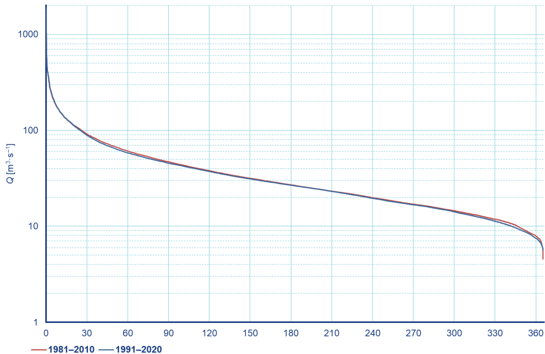
Obr. 6. Čáry překročení M -denních průtoků v období 1981–2010 a v období 1991–2020 v profilu vodoměrné stanice Bohumín na Odře
